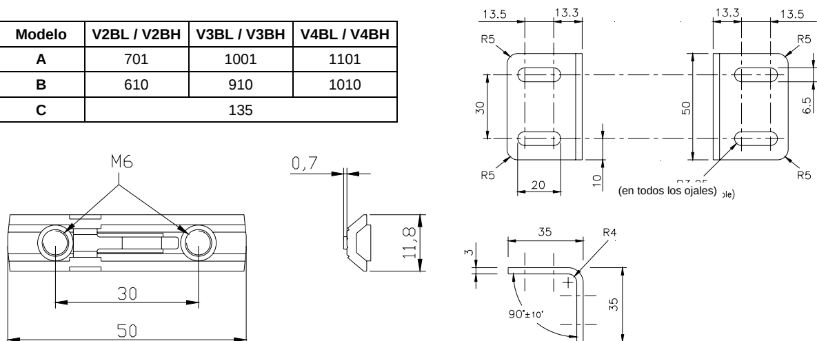
Figura 19 Adaptadores y escuadras de fijación (suministradas)
