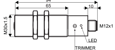
VISTA PARTE SENSIBILE SENSITIVE SIDE VIEW
