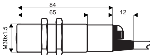
VISTA PARTE SENSIBILE SENSITIVE SIDE VIEW
