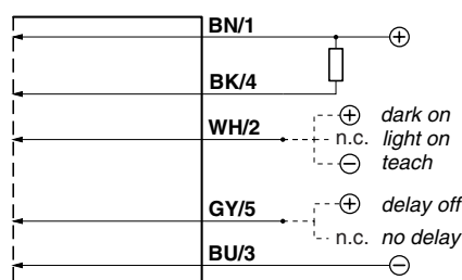
NPN uscita/output
