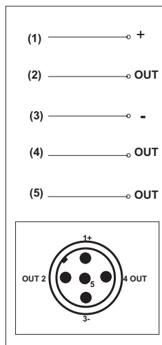
CA - CB 5 POLI/ 5 WIRES
