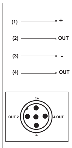
CA - CB 4 POLI/ 4 WIRES
