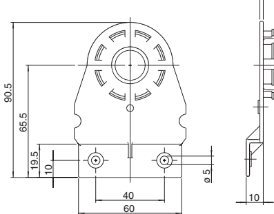
Pletina de montaje 6482
