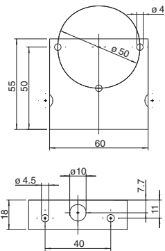
Pletina de montaje 6401
