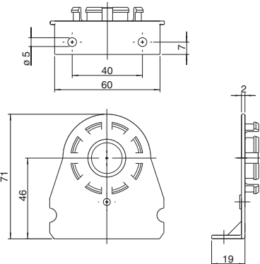
Pletina de montaje 6481
